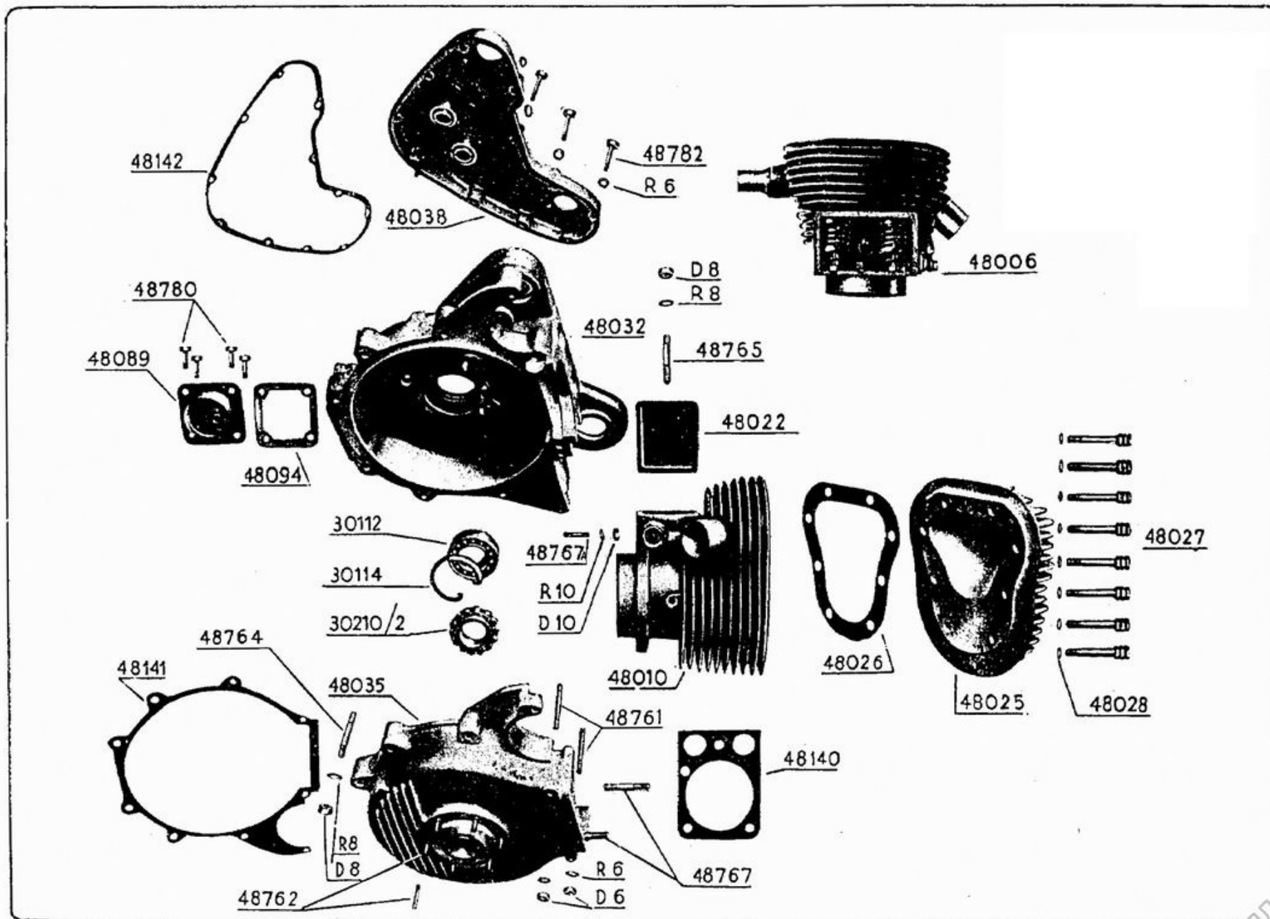
Testa - cilindro - carter - coperchi
