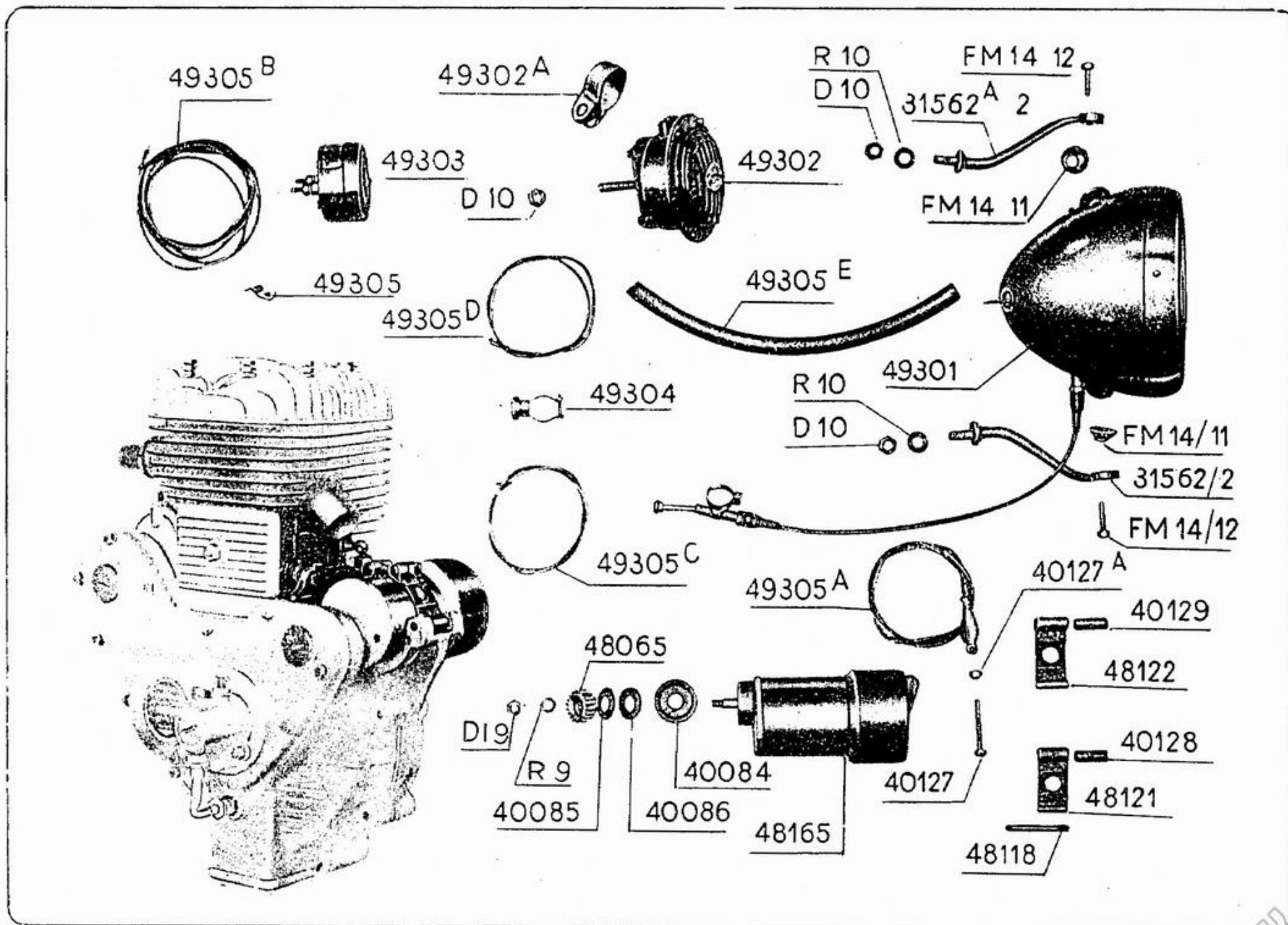
Dinamo - fero - avvisatore elettrico
