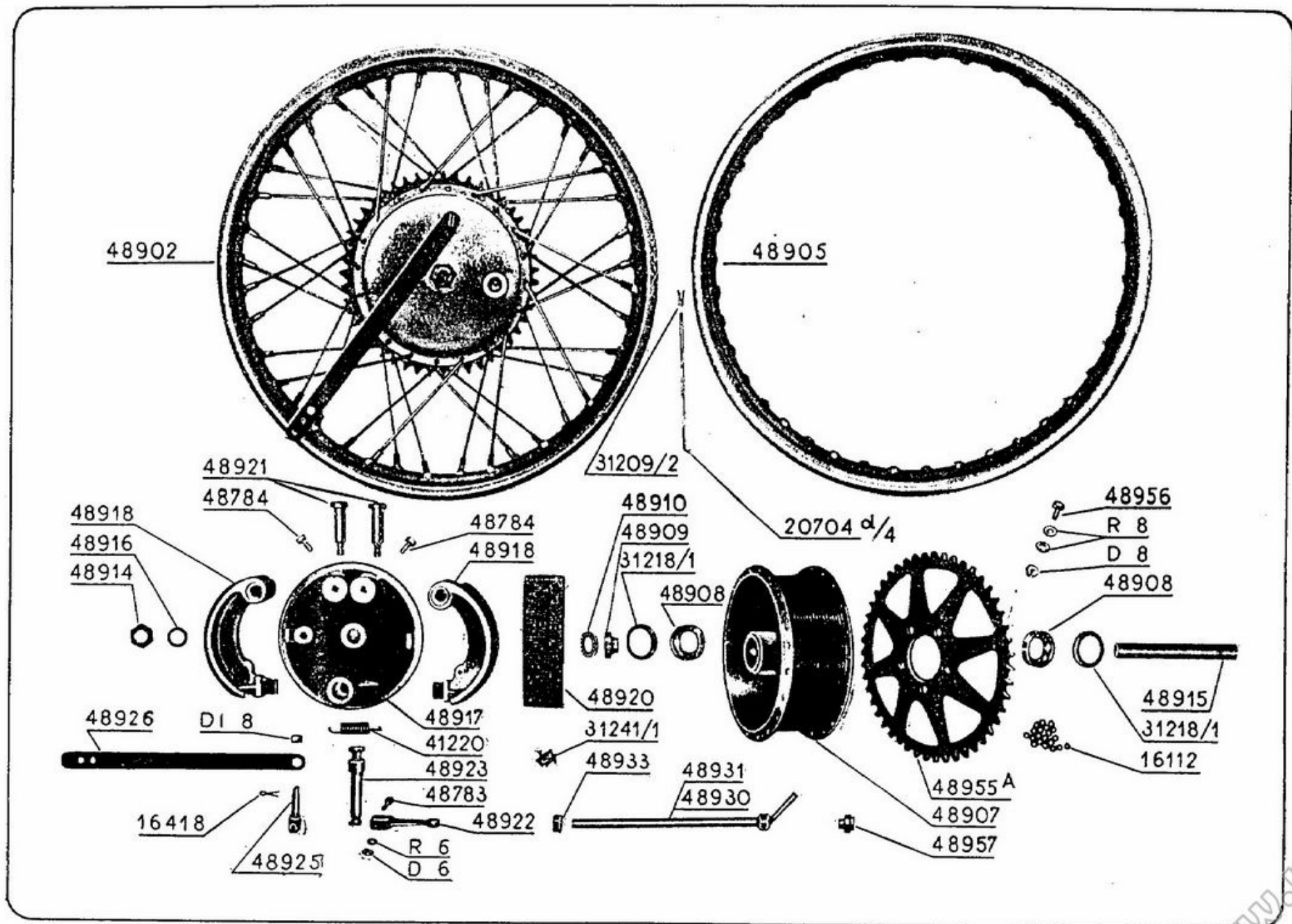
Ruola - mozzo - freno
