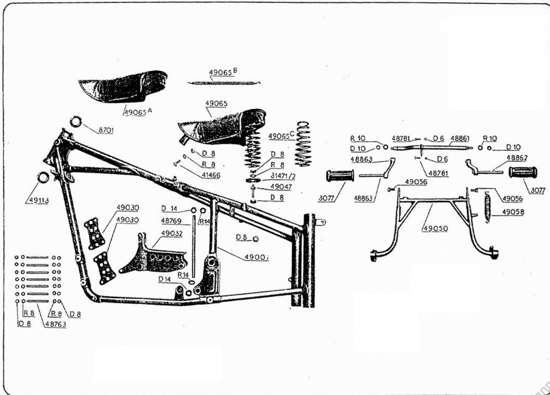
Telaio - sella
