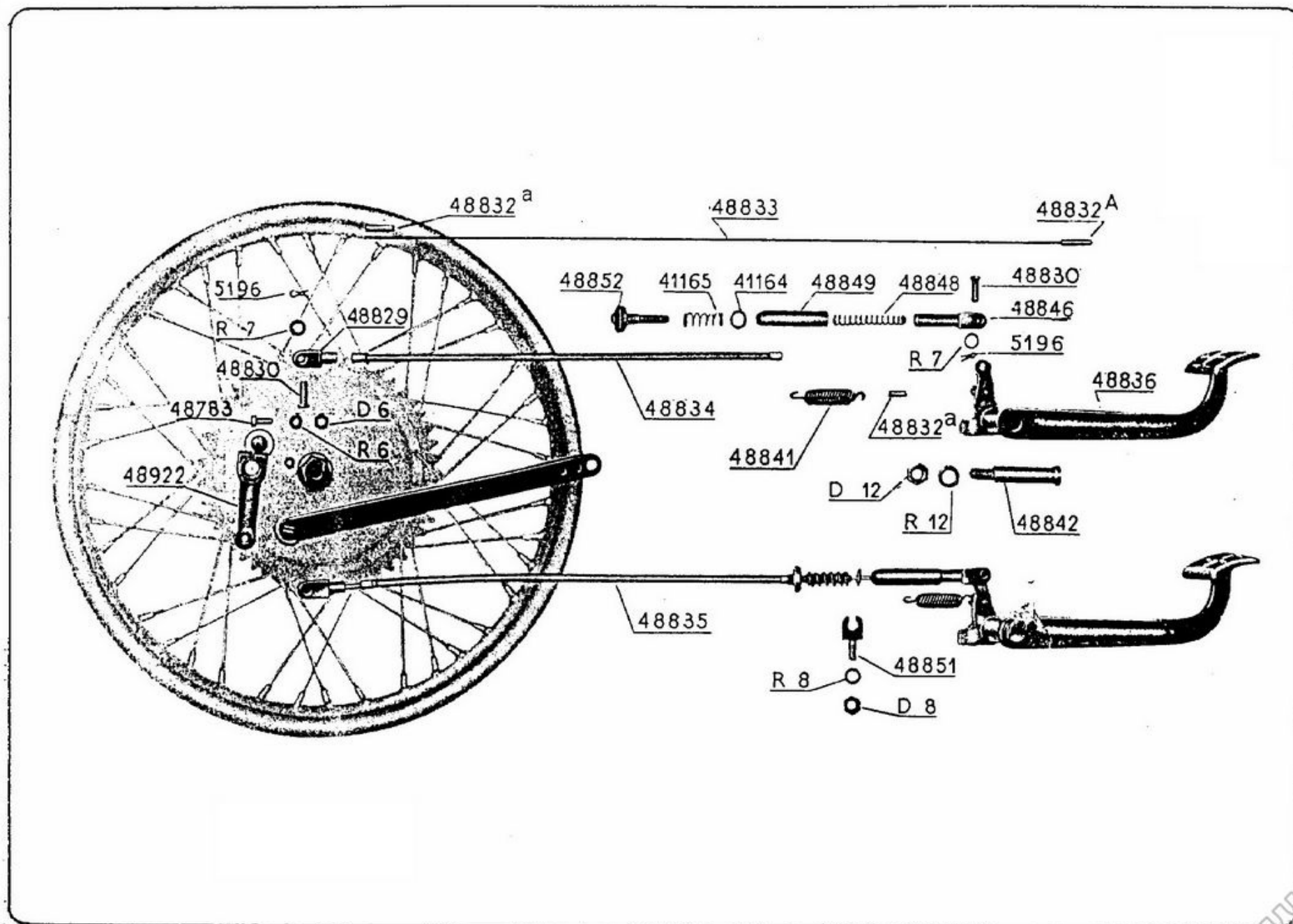
Comando freno posteriore
