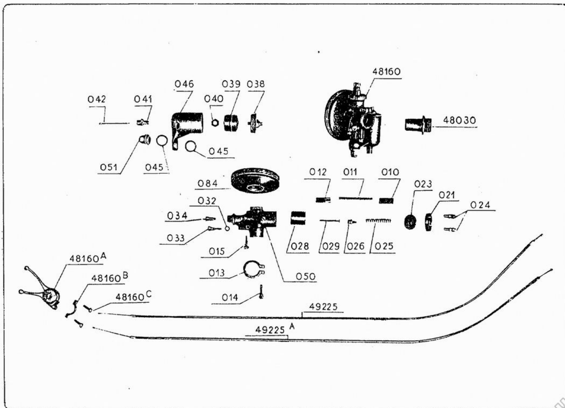
Parti del carburatore
