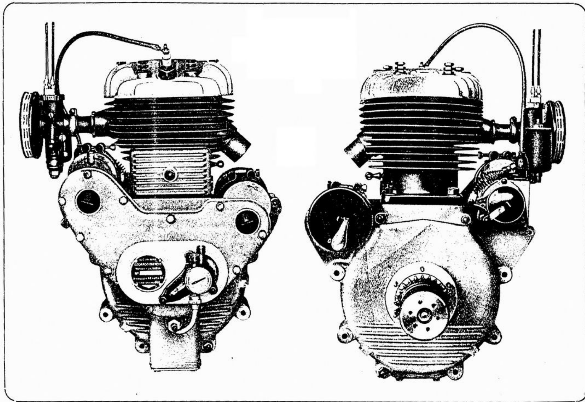
Motore BIANCHI 500 cmc.
