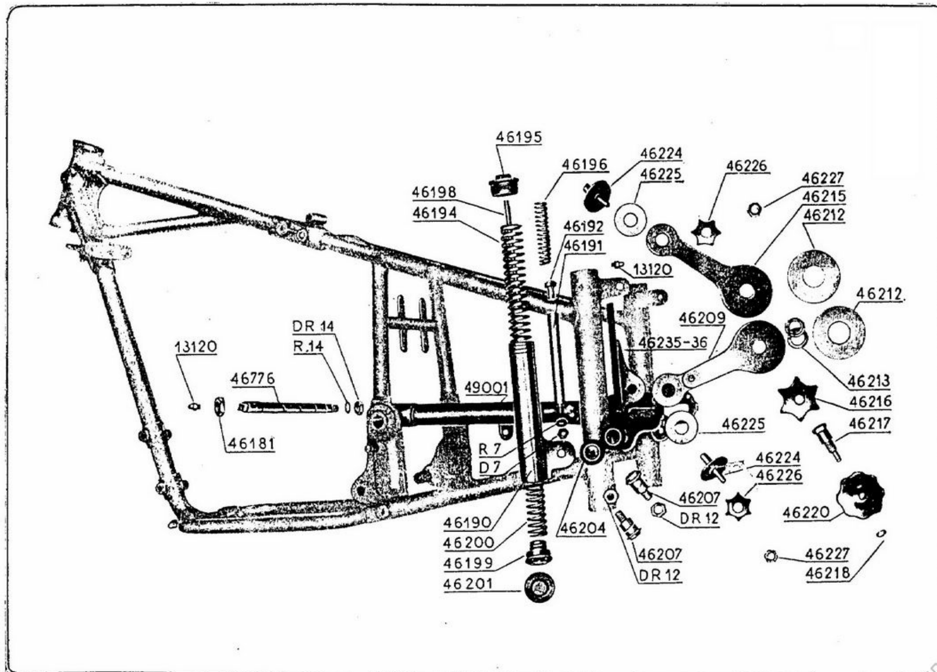
Sospensione elastica posteriore
