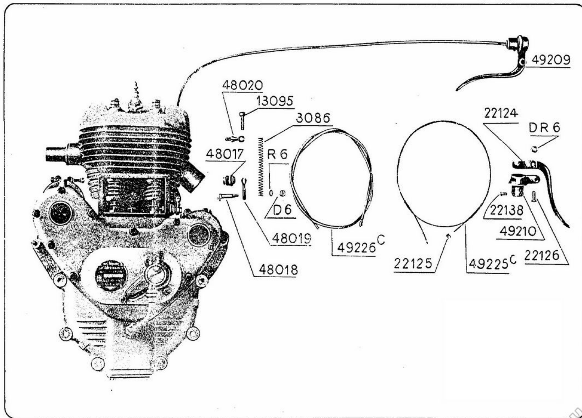
Alza valvola
