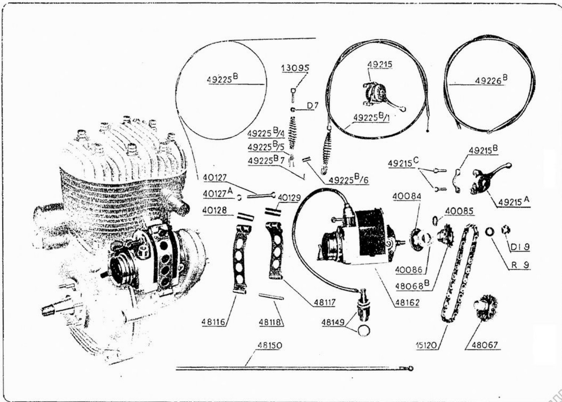
Магнете
