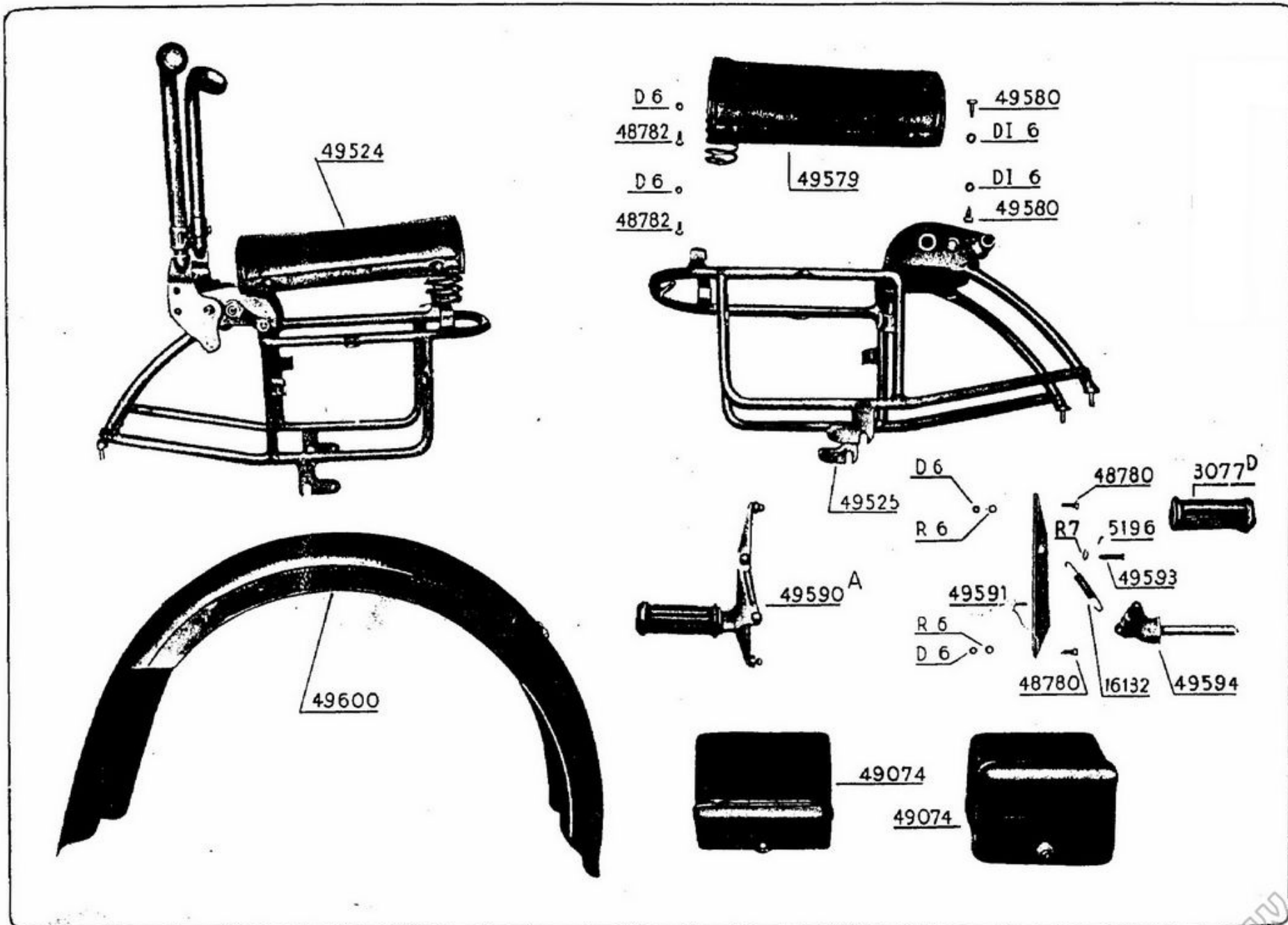
Supporto sellino posteriore - appoggiapiedi - parafrango
