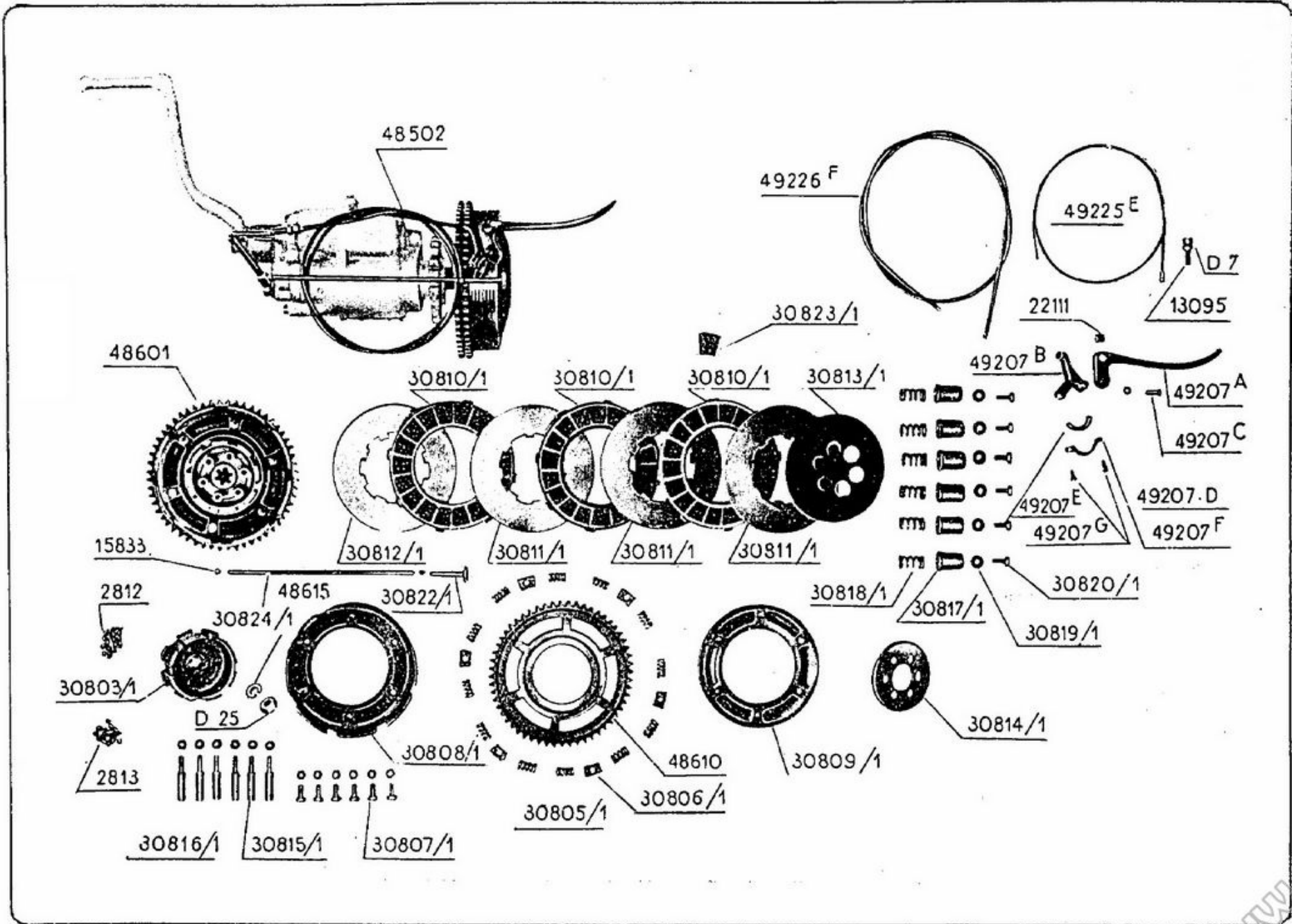
Frizione
