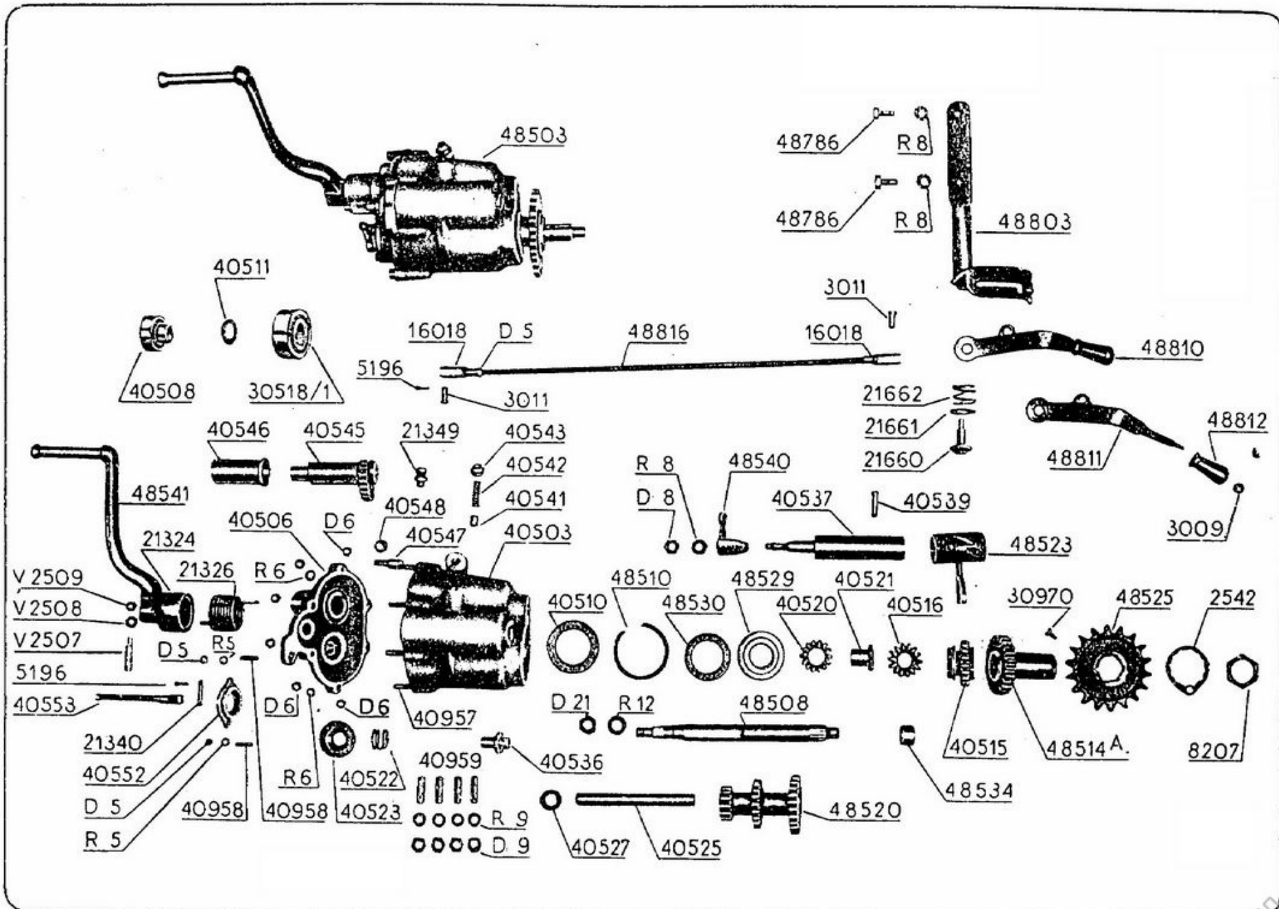
Cambio di velocità e comando
