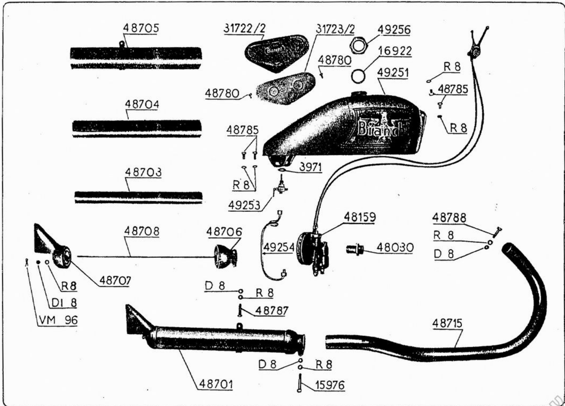
Serbatoio - carburatore - silenziatore
