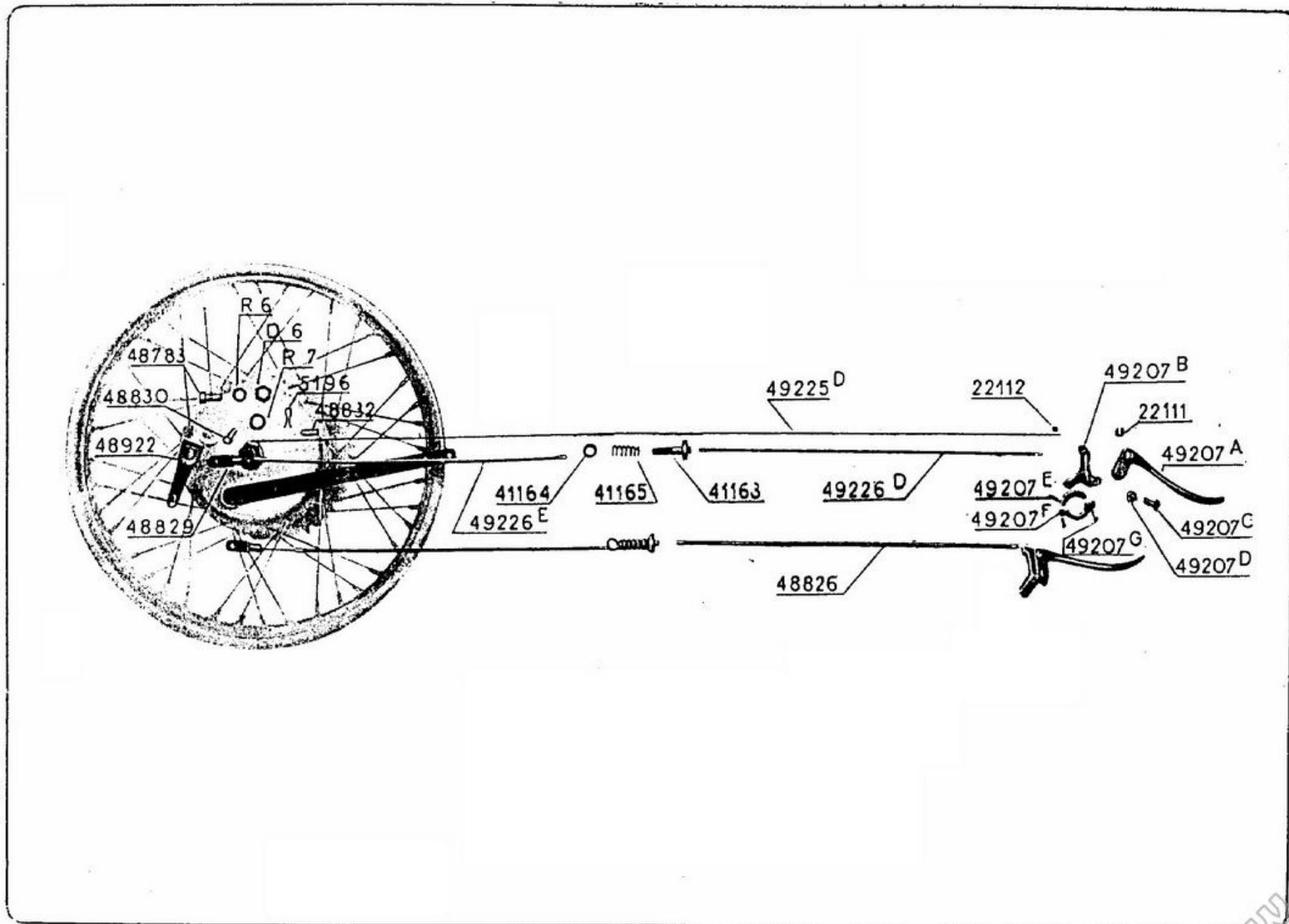
Comando freno anteriore
