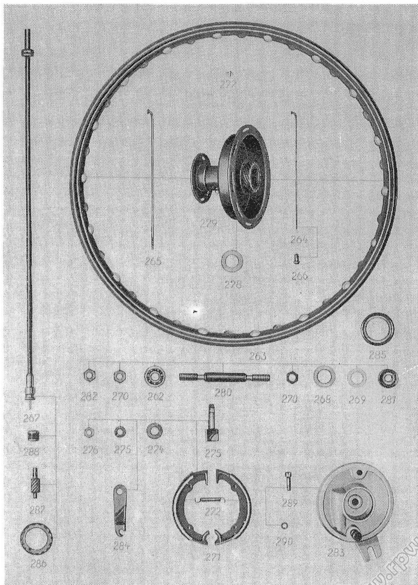
Tafel 12, Gruppe B: a) Vorderrad mit Bremse, Geschwindigkeitsmesserantrieb
