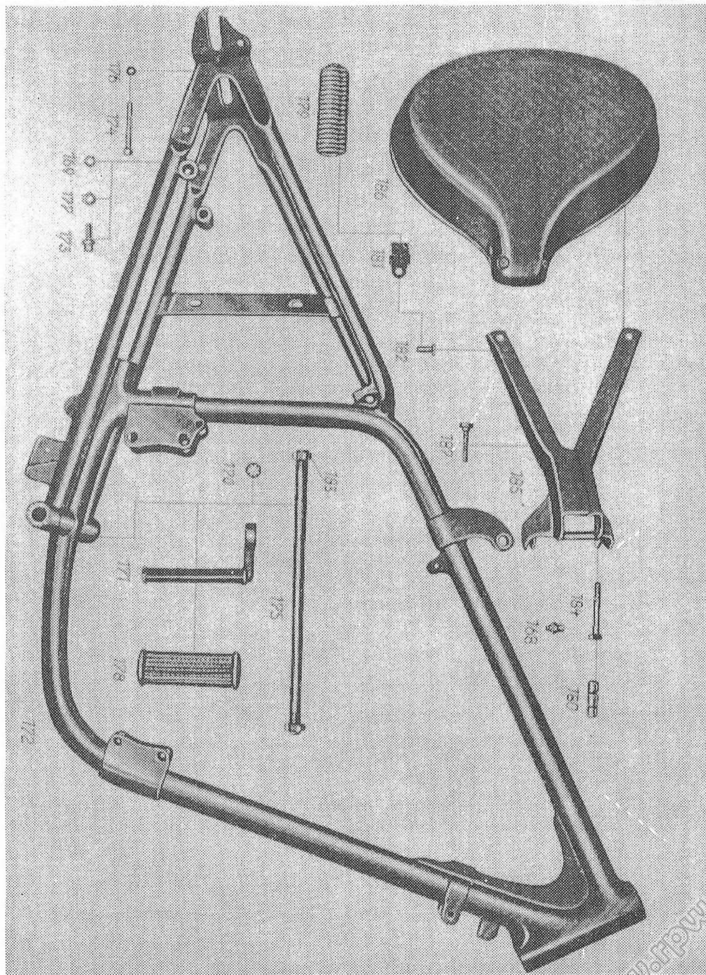
Tafel 7, Gruppe R: a) Rahmen, Fußraster, Sattel
