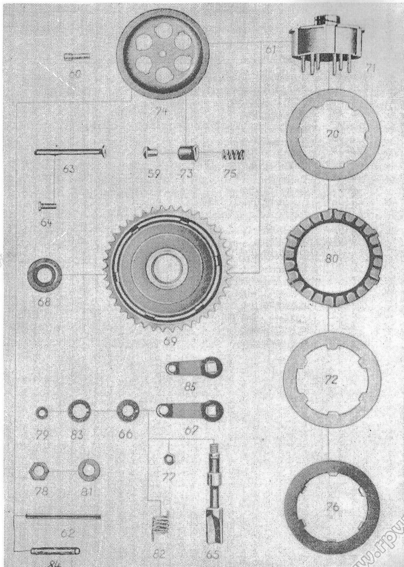
Tafel 4, Gruppe M: d) Mehrscheibenkupplung
