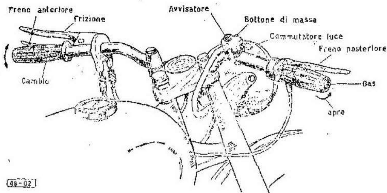
Fig. 2 - Manubrio e comandi
