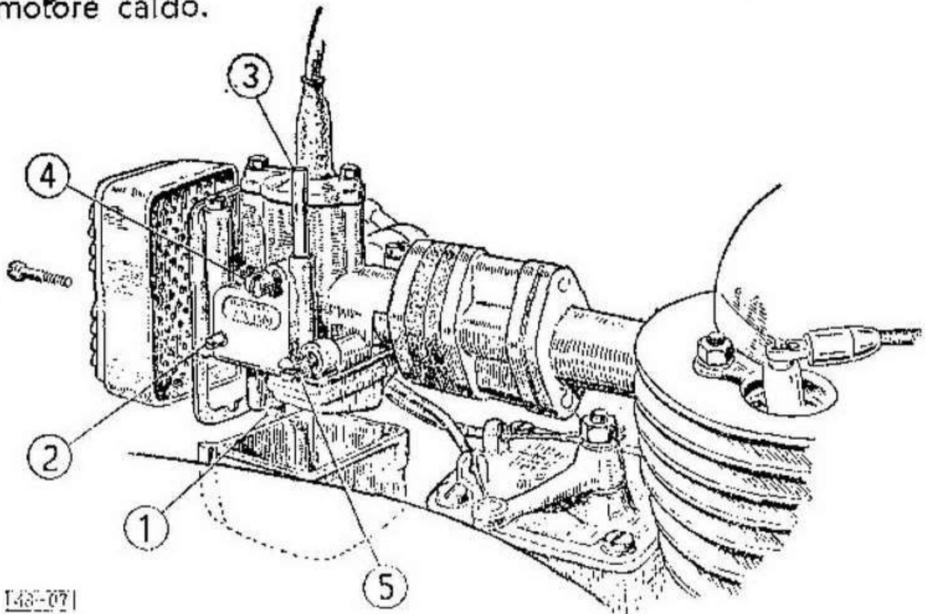
Fig. 7 - Carburatore « Dell'Orto » SH 14/9
