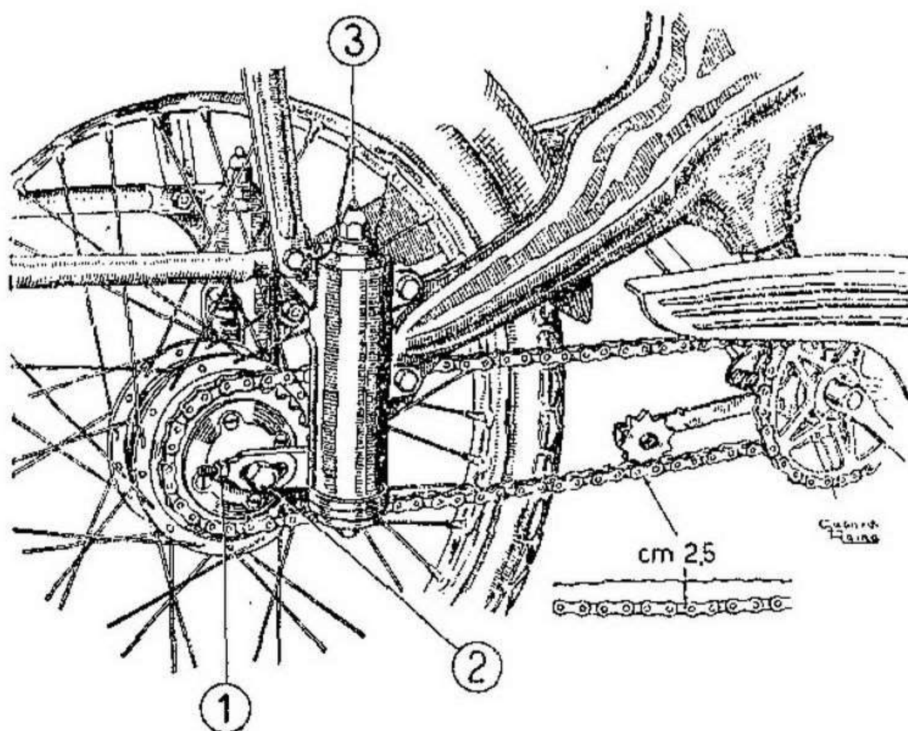
Fig. 12 - Regolazione tensione catena - Sospensione posteriore
