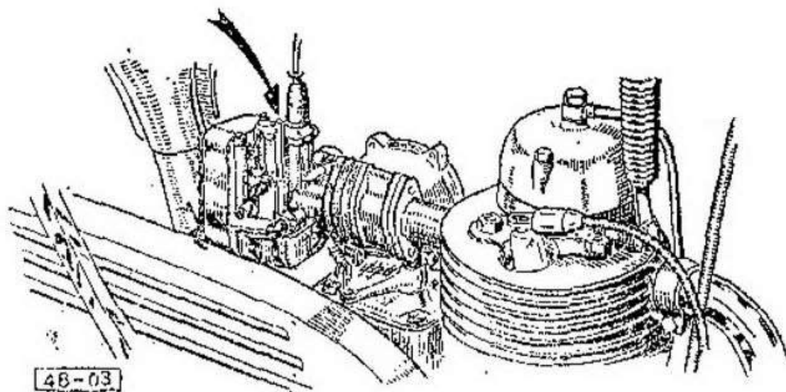
Fig. 3 - Agitatore del galleggiante sul carburatore « Dell'Orto »
