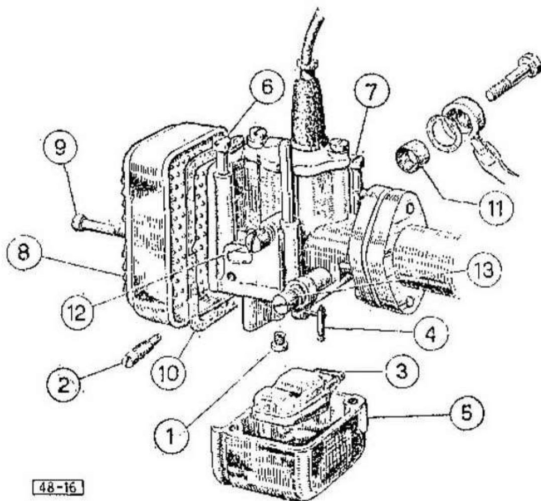
Fig. 15 - Pulizia carburatore « Dell'Orto »
