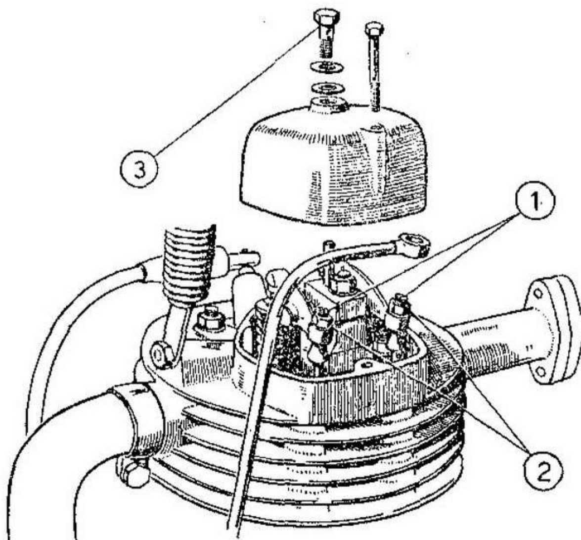
Fig. 8 - Regolazione giuoco comando valvole
