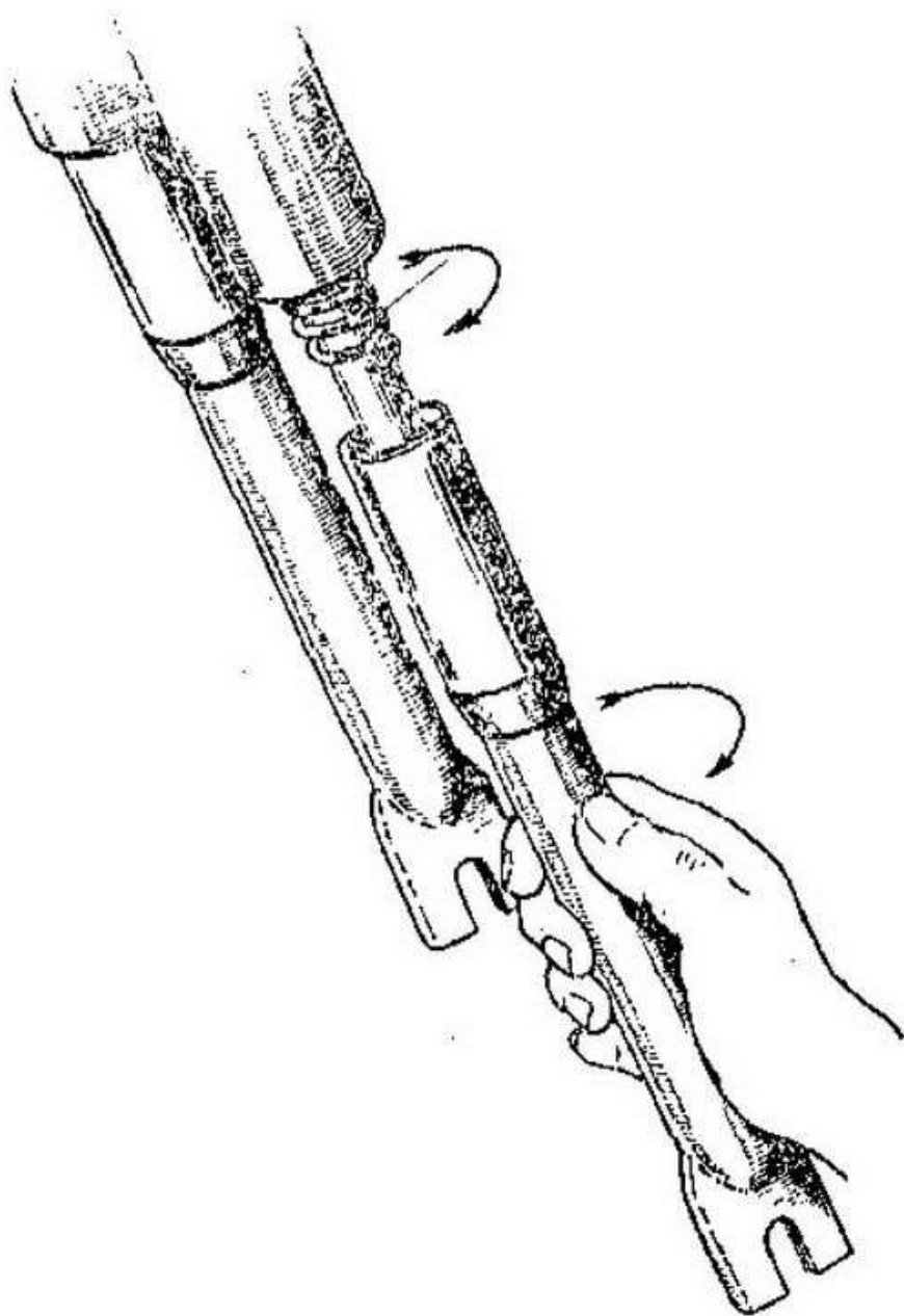
Fig. 6 - Smontaggio della forcella telescopica
