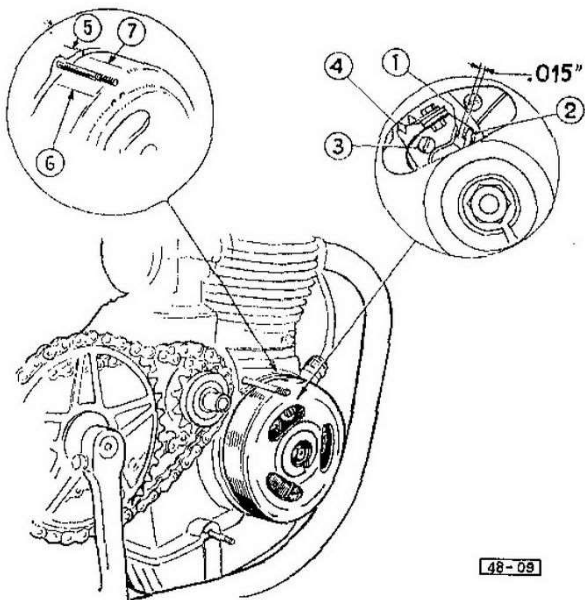
Fig. 9 - Regolazione contatti del rottore
