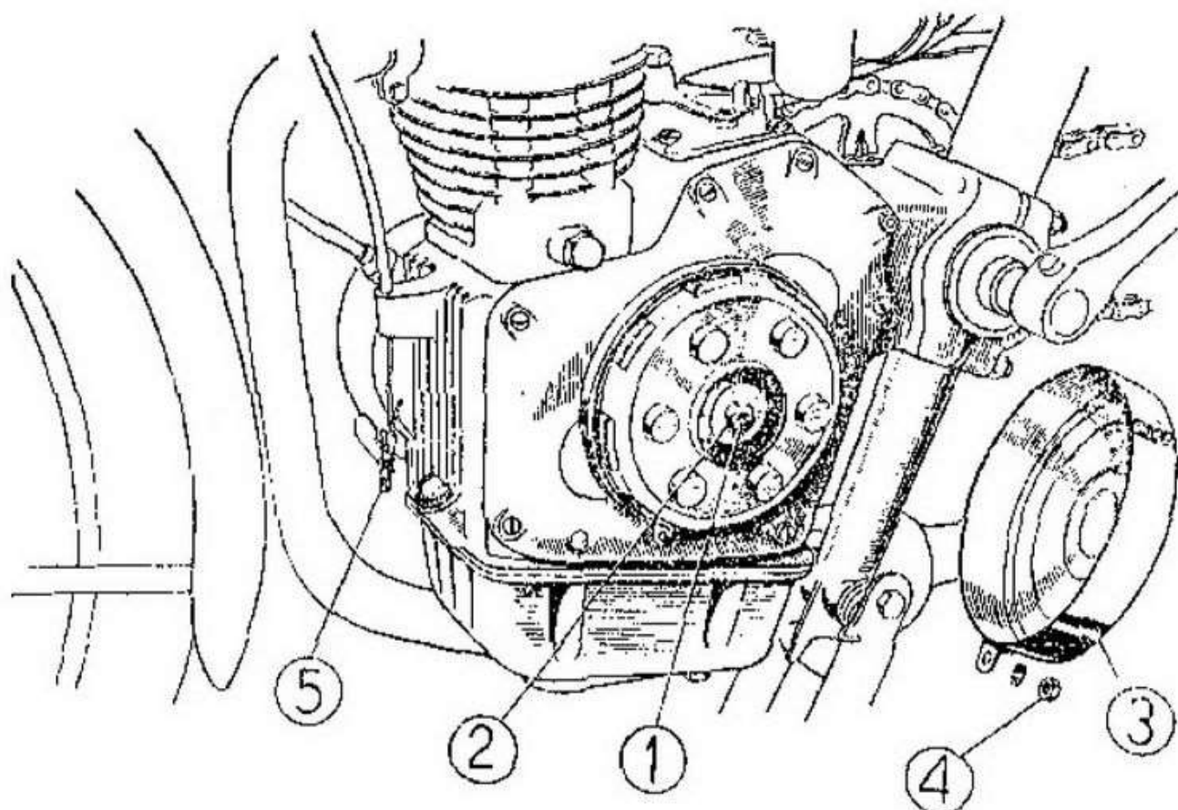
Fig. 10 - Regolazione giuoco comando frizione
