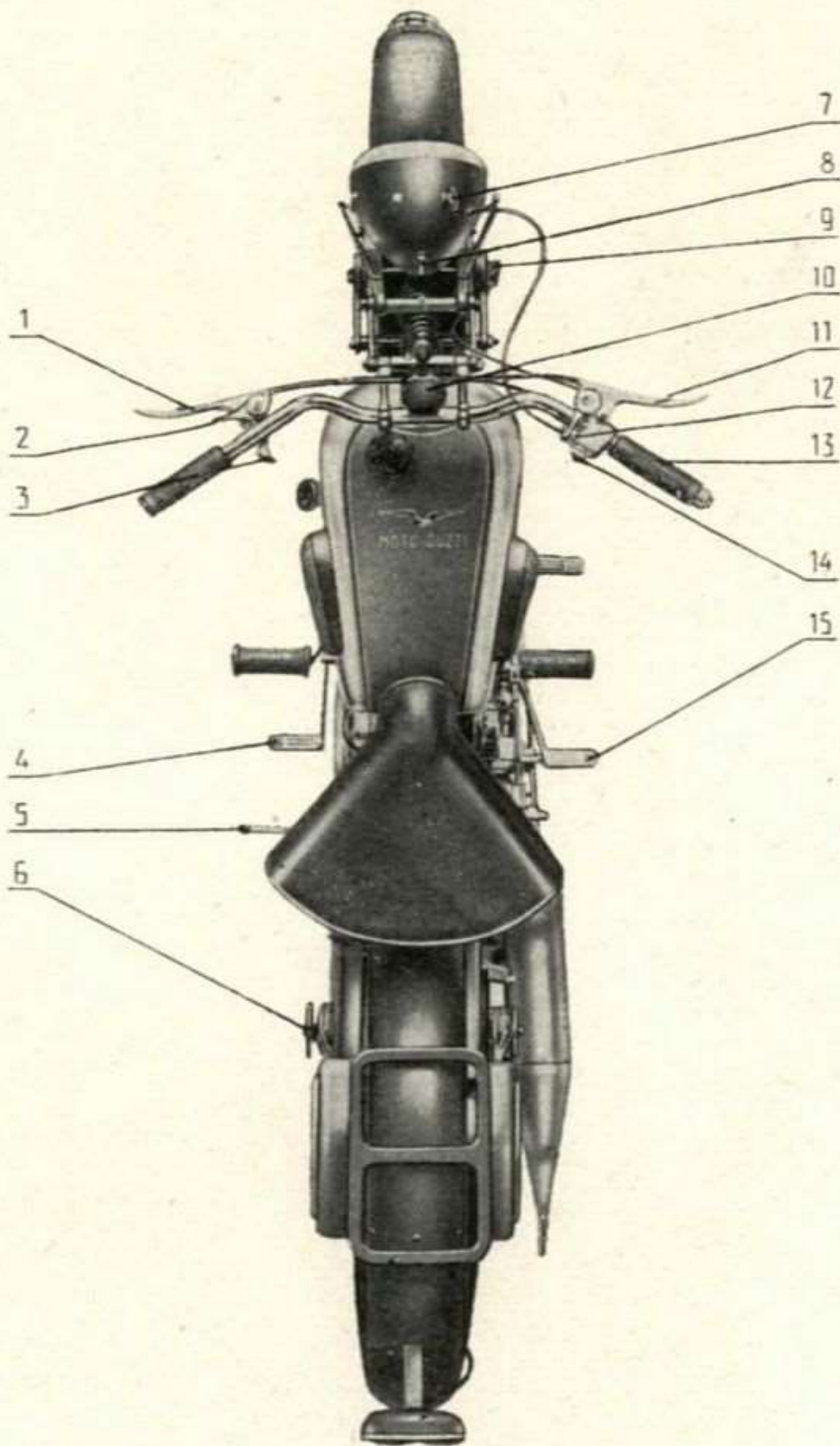
Fig. 3 — Motociclo AIRONE ( comandi )
